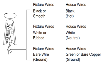
Fig. 2 Wiring
